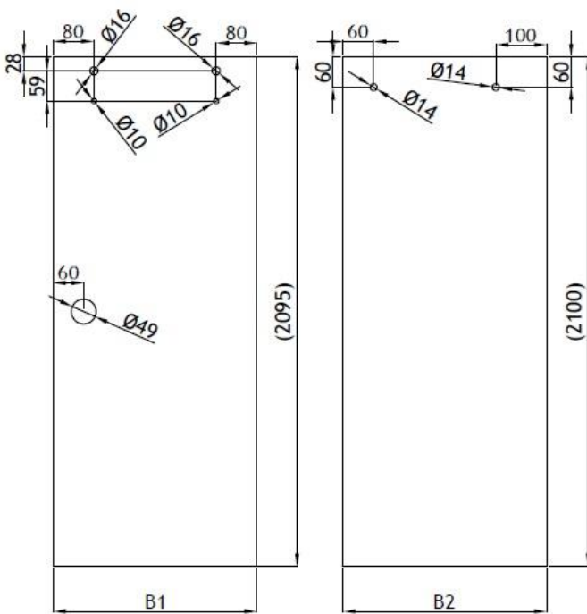
Schiebetür
