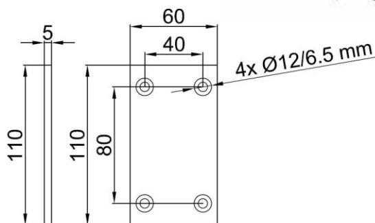
Anschraubplatte:
