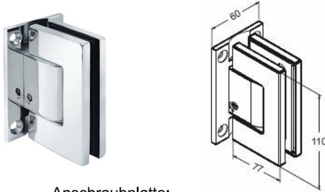
Anschraubplatte:
